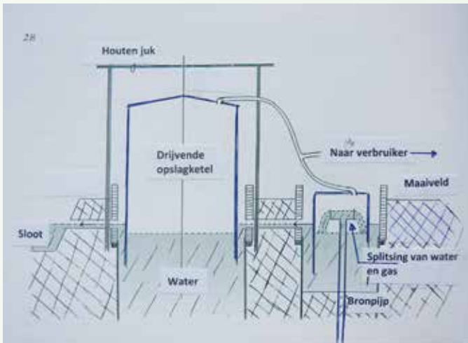
Schematische weergave brongasinstallatie
